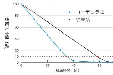
速乾性 (拡散性残留水分率)
